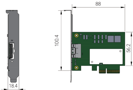
PCIe-SAS441
